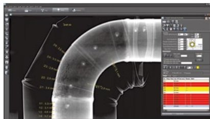
Wanddickenmessung
